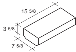
8x4x16 Beveled Cap
