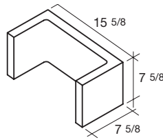
16x8x8 C-Alternate
